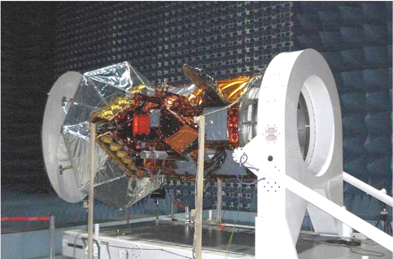
SAC-D en la cámara anecoide del INPE/LIT, un recinto con paredes que lo aíslan de toda energía electromagnética, tal como se encontrará en el espacio.
